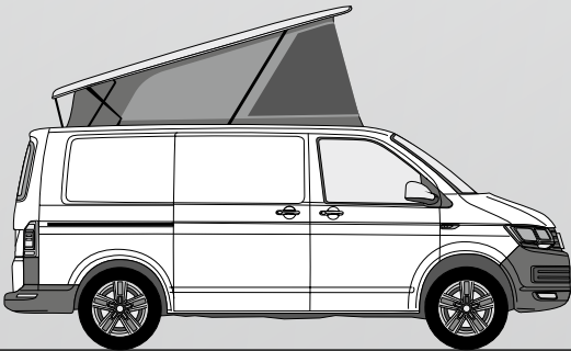
SCA 290: Aufstellart vorne für Radstand 3.000mm (kurze Version)
